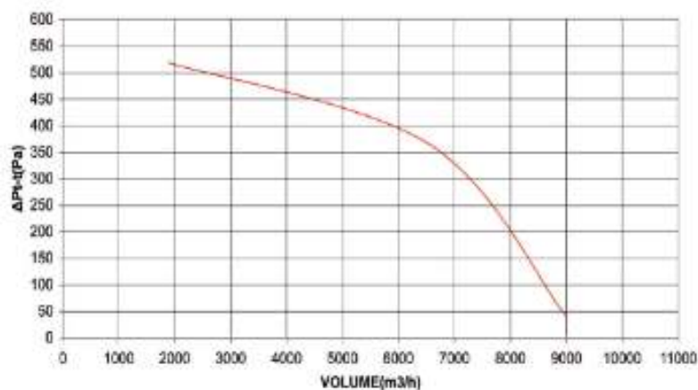
Φ350-3.0HP-1450RPM
