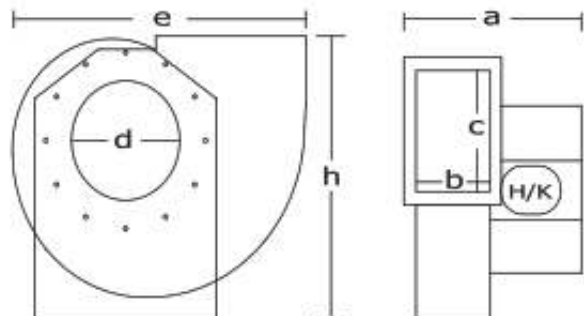
Φ350-3.0HP-1450RPM
